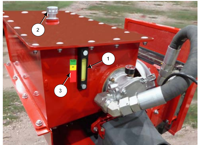
Replace the Filler Cap
