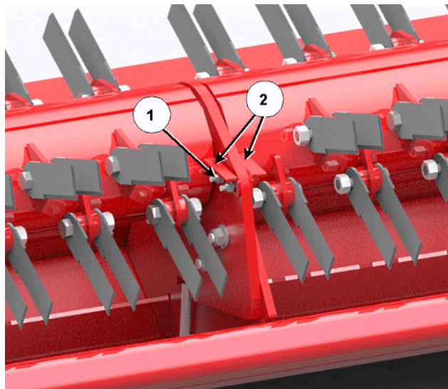
Отрегулируйте шпигатные скребки – центральной опорной плиты
