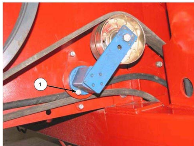
Регулировка натяжения ремня
