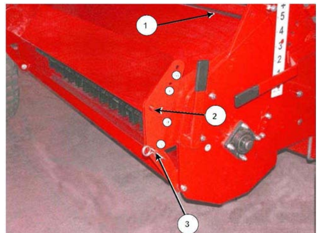
Установки разгрузочной дверцы для измельчения корма
