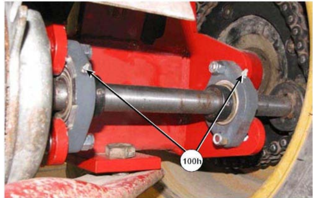
Смазывайте подшипники вала муфты
