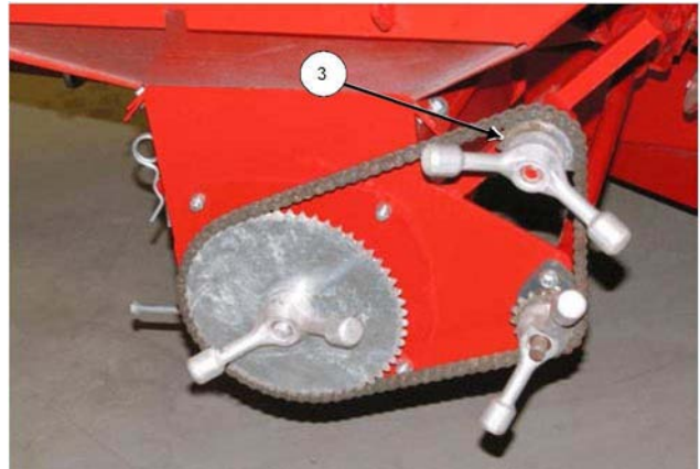
Ослабьте цепь
