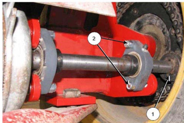
Отрегулируйте положение звездочки приводного вала
