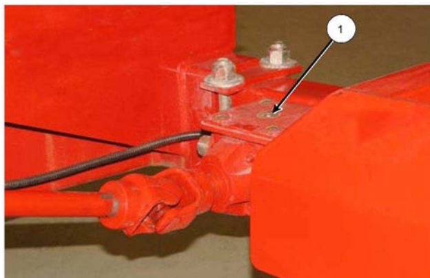
Нижний редуктор (снять держатель ведра и трубку) 211184C
