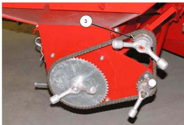
Ослабьте цепь
