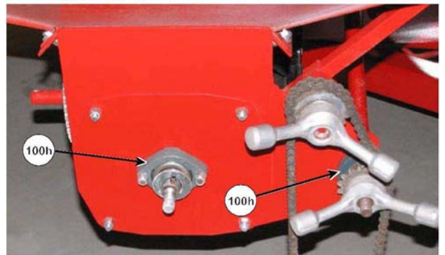
Смазывайте подшипники шнека и его привода
