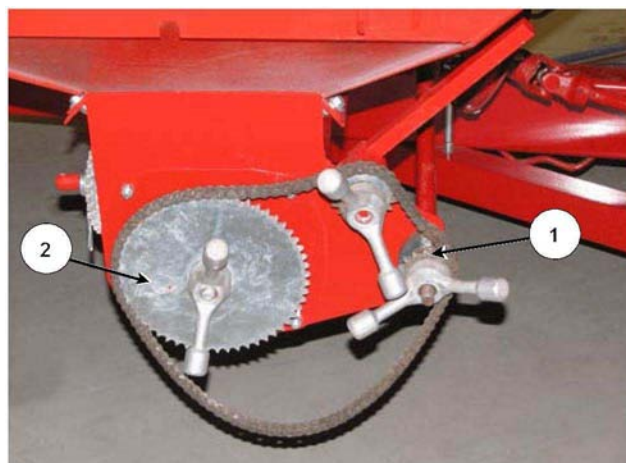
Установите ведущую звездочку и звездочку шнека
