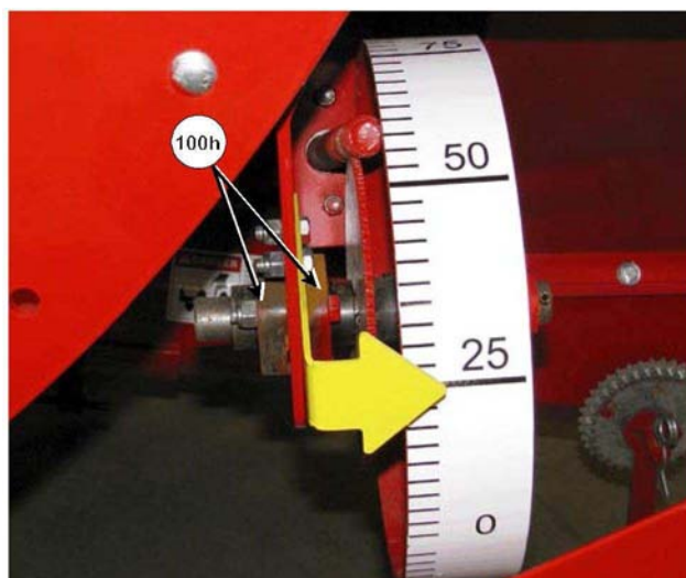
Смазывайте двусторонние подшипники счетчика длины пути
