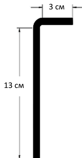
Измеритель уровня масла 212056
