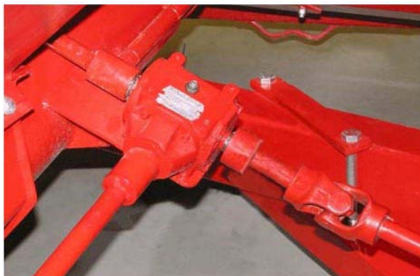
Верхний редуктор (снять трубку сапуна)
