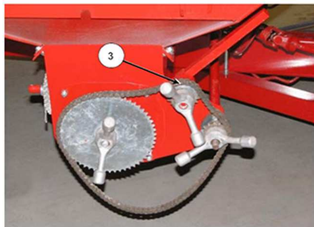
Ослабьте и снимите приводную цепь
